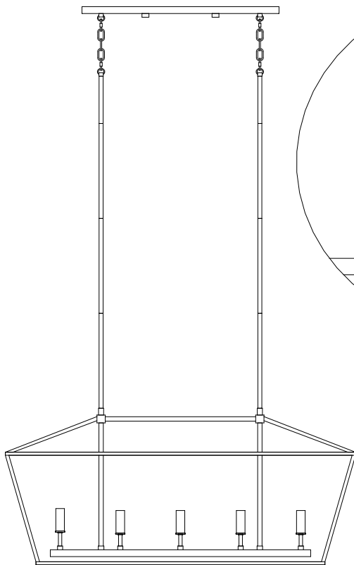
5-LIGHT PENDANT
